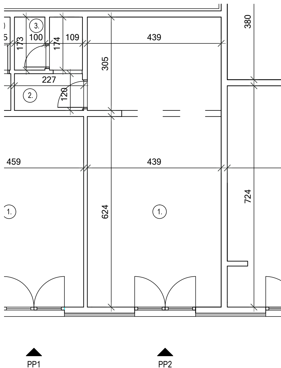
TLOCRT POSLOVNOG PROSTORA
