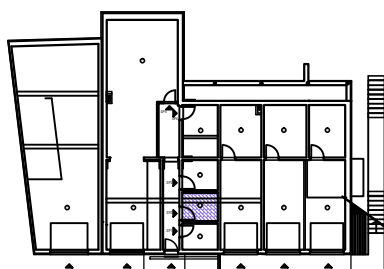
TLOCRT PODRUMA
