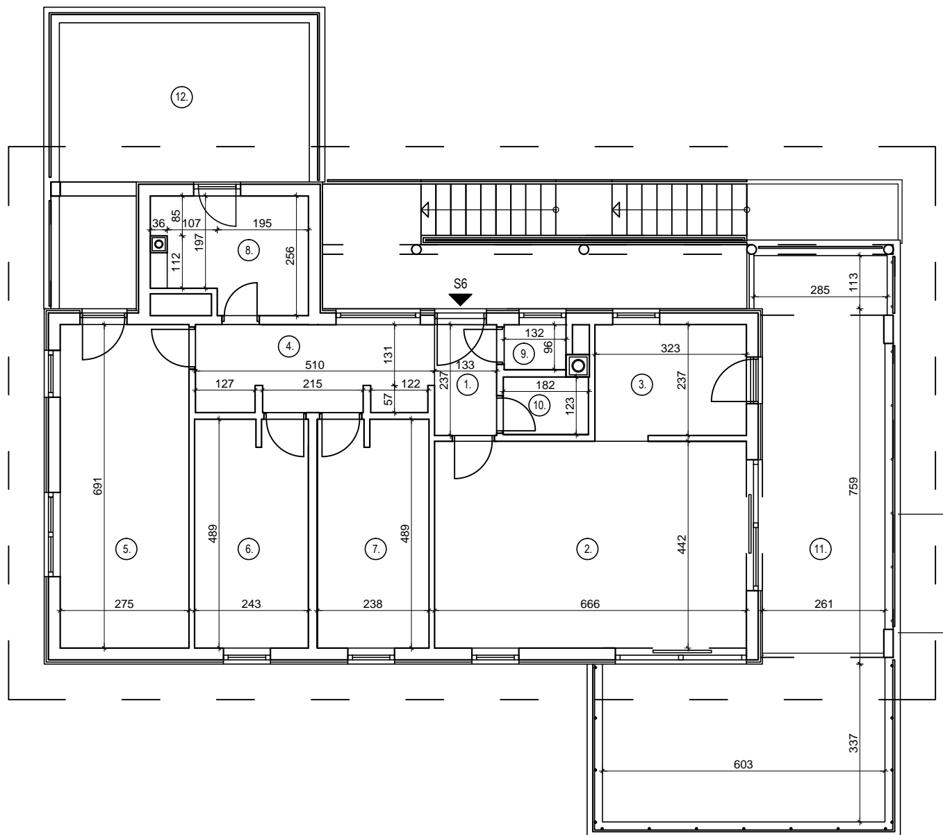
TLOCRT STANA
